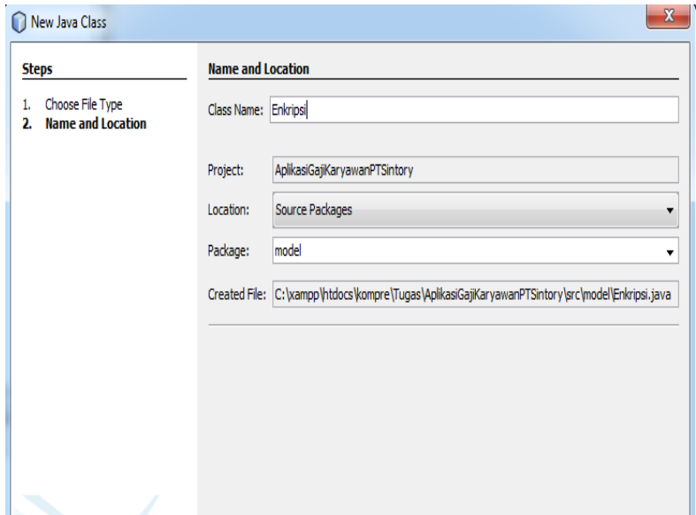
Gambar 5. 7 Membuat Enkripsi
