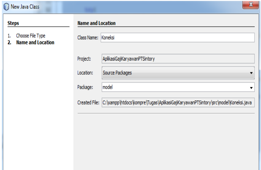
Gambar 6. 1 Membuat Koneksi
