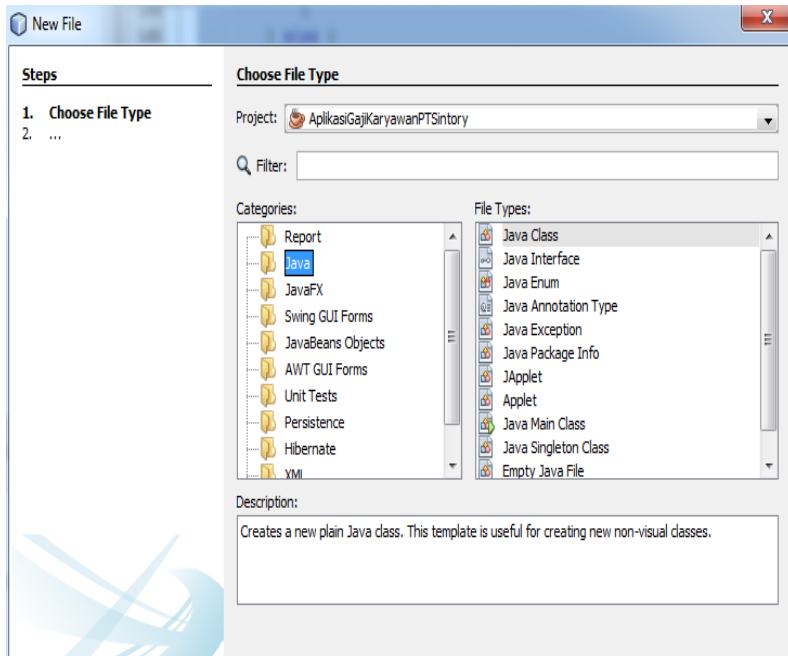
Gambar 5. 1 Membuat Class
